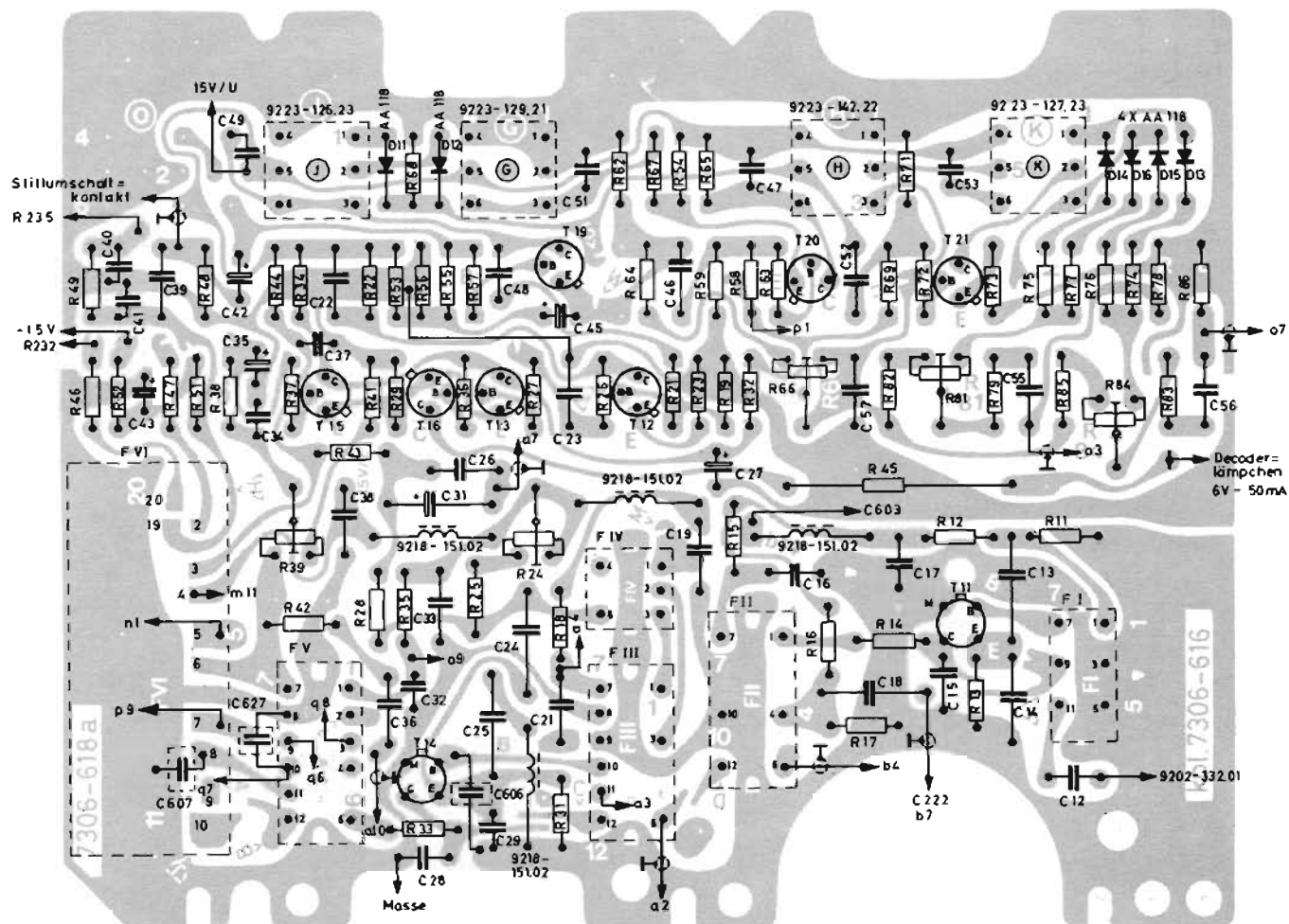
PLATINE FI/ AM-FM, VUE DU COTE DES COMPOSANTS
