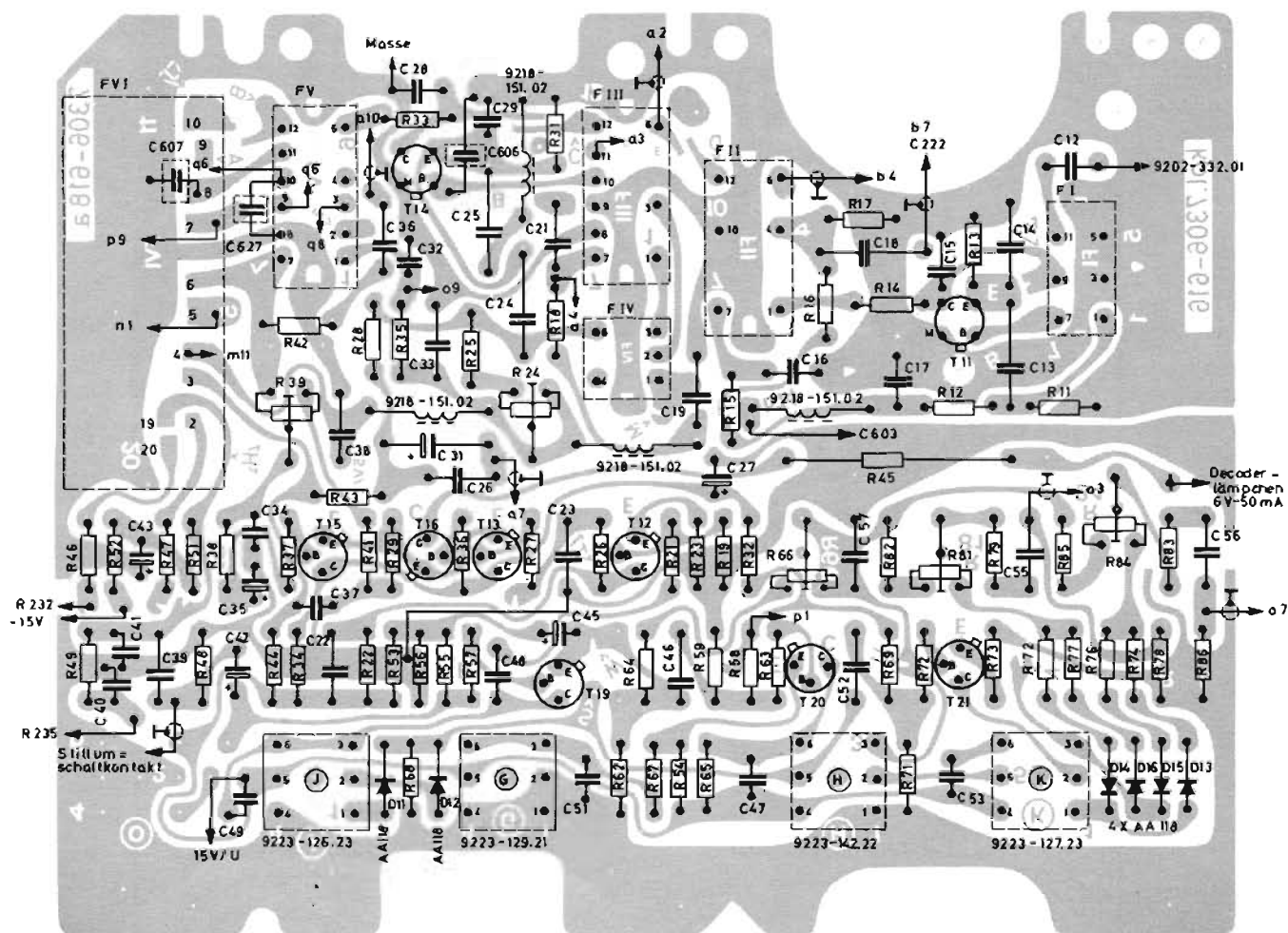
PLATINE FI/ AM-FM, VUE DU COTE DES COMPOSANTS
