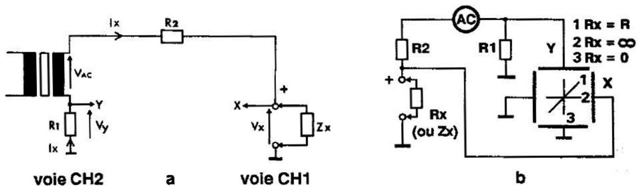
Branchement du composant Z_x
