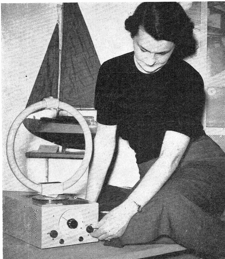
Cet original récepteur portable anglais à cadre est prévu pour permettre la navigation ; il peut, en effet, recevoir les signaux des radio-phares et donne des positions à l'intérieur d'un champ de 2° jusqu'à 50 miles.
