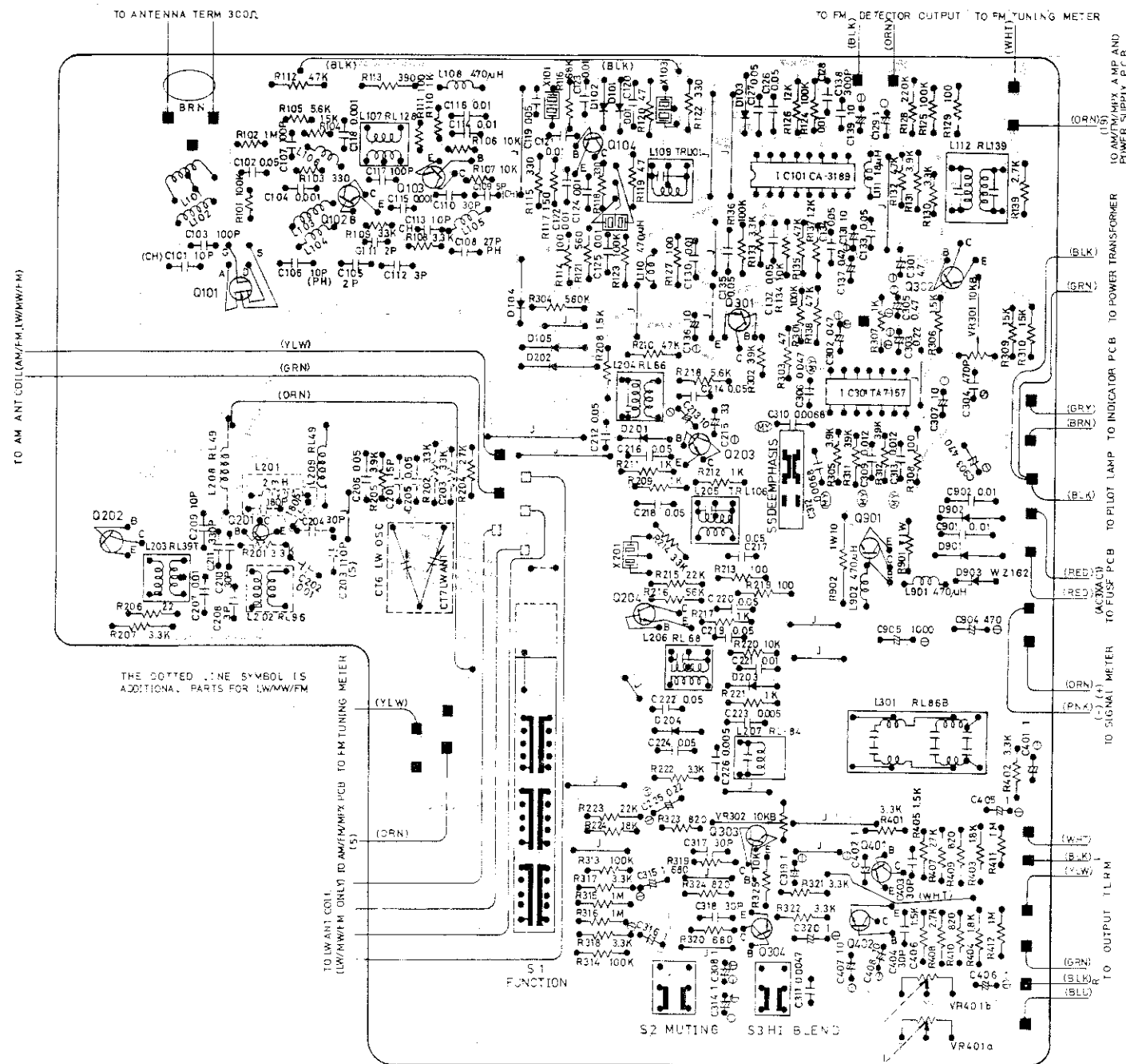
AM/FM/MPX Amp. Circuit Board Diagram Schaltbild des AM/UKW/MPX Vertäekers und Vorverstäekers (RT-726) Diagramme de Plaque du Circuit d'Amp. AM/FM/MPX
