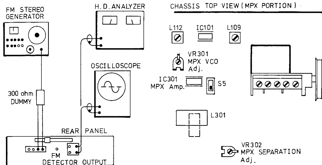
Fig. 5. FM MPX Alignment Hook-Up Abb. 5. UKW-MPX-Einstellung Fig. 5. Alignement FM MPX
