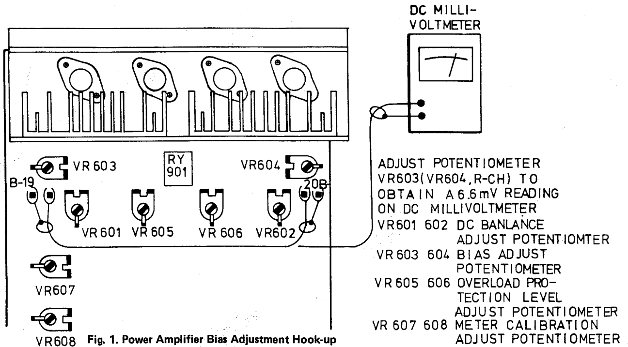
Abb. 1. Messanschluss zur Endverstaerker Ker-Vorspannungs-Einstellung
