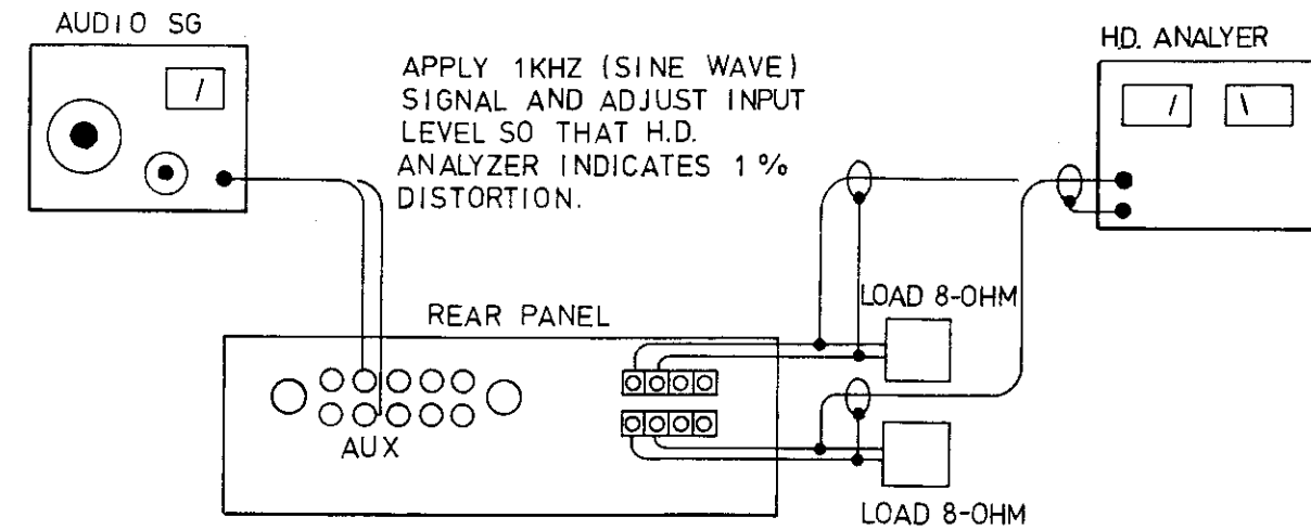
Fig. 3. Overload Protection Level Adjustment Hook-up Abb. 3. Ueberlastungsschutzpegel-Einstellung Ahgleich Fig. 3. Réglage du Niveau de la Protection de Surchage
