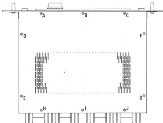
Fig. 1-1 TOPVIEW
