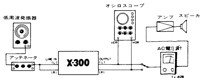
図 2-3 接続図
