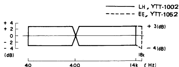
図 2-7 再生周波数特性 (LOW)
