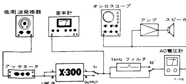
図 2-2 接続図
