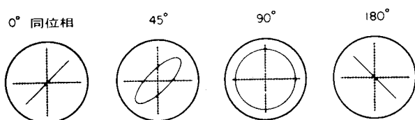
図 2-4 位相の確認
