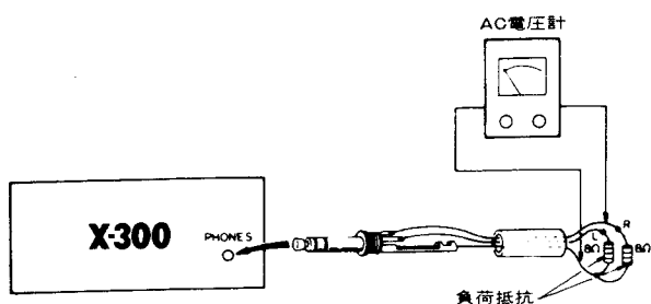
図 2-5 接続図
