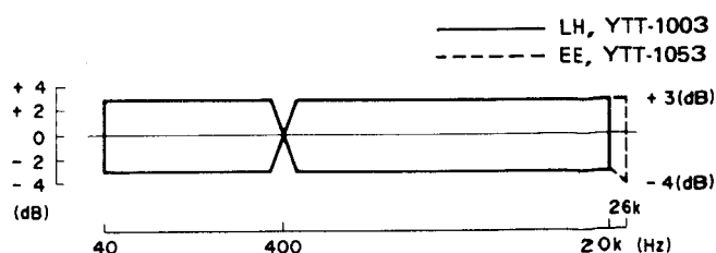
図 2-6 再生周波数特性 (HIGH)
