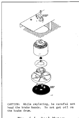
Fig. 4-4 Reel Motor
