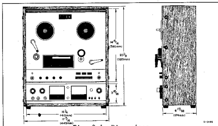
Fig. 2-1 Dimensions
