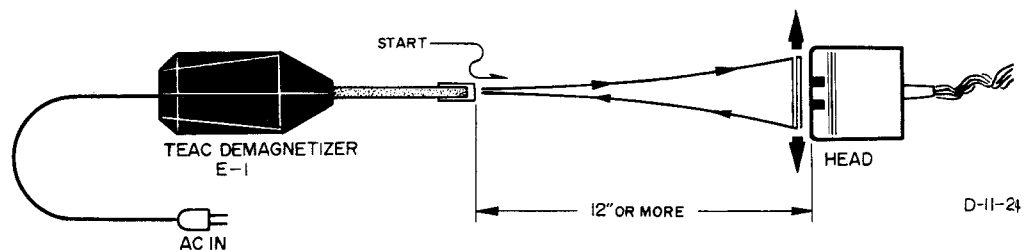
Fig. 8-2 Demagnetization
