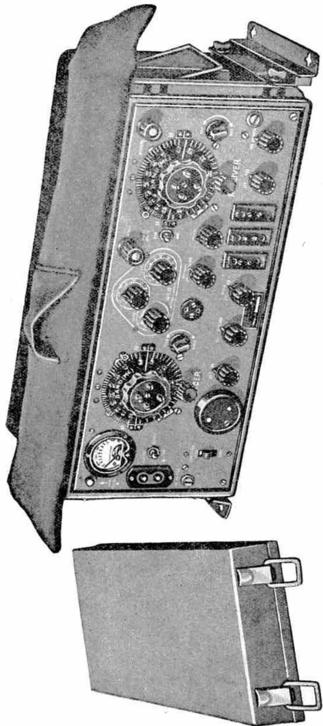
FIG.1 VUE GÉNÉRALE DU POSTE MONTÉ SUR SUPPORTS ÉLASTIQUES
