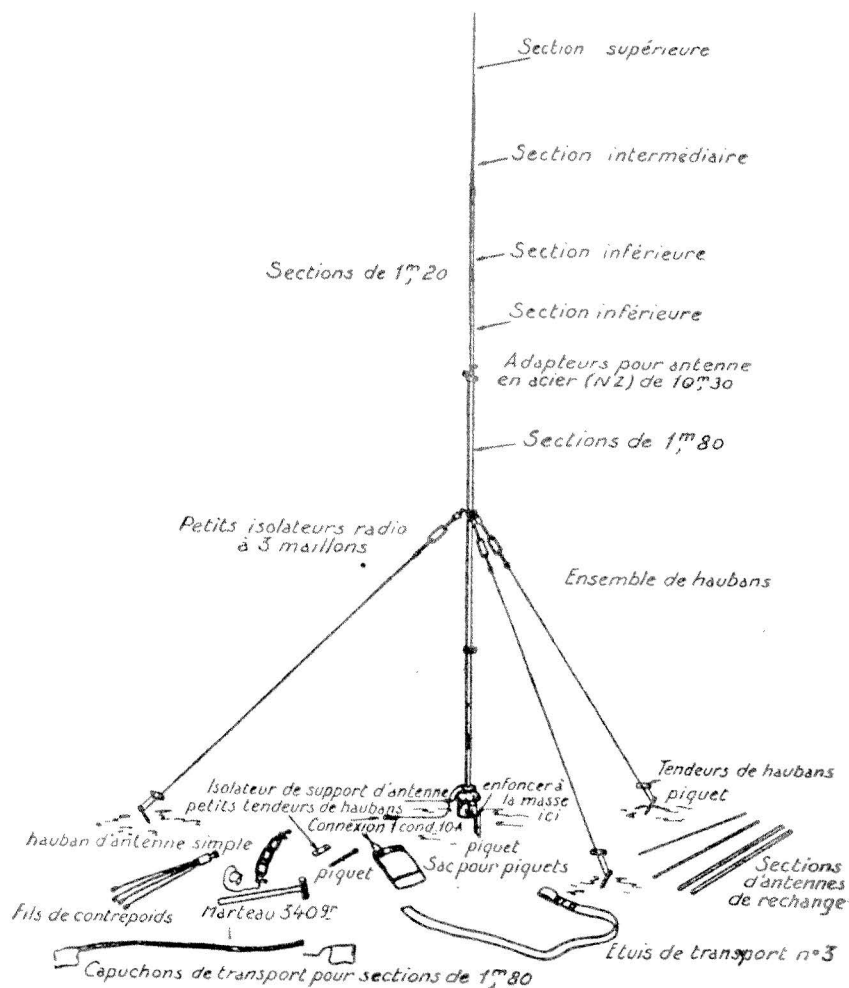
FIG. 3 MONTAGE DES ANTENNES DE 10m,30
