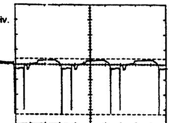
OSZ-12 5,9 Vss, 20 µs/Div. H-Flyback
