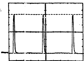
OSZ-18 27 Vss, 5 ms/Div. TDA 8170 Pin 3
