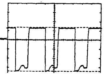
OSZ-8 2,4 Vss, 20 µs/Div. T 301 Basis
