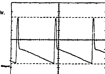
OSZ-17 3,5 Vss, 5 ms/Div. TDA 8170 Pin 3
