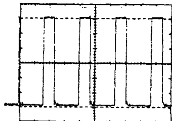
OSZ-1* 12 Vss, 5 µs/Div. TDA 4605 Pin 5
