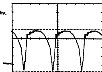
OSZ-13b 16,5 Vss, 5 ms/Div. TR 302 Pin 7
