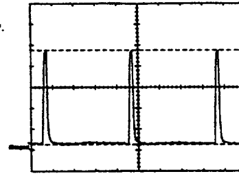
OSZ-20 4,5 Vss, 5 ms/Div. CR 409/CR 410
