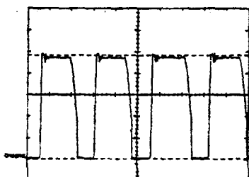
OSZ-2* 480 Vss, 5 µs/Div. T 101 Drain
