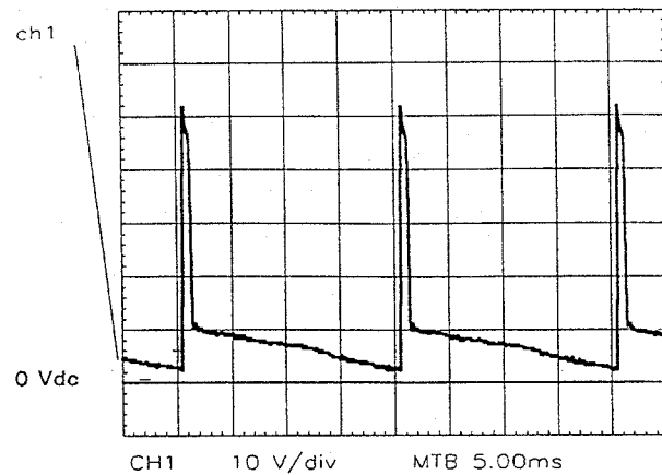
Pin 9 IC601
