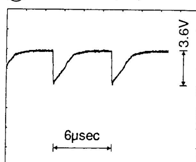
⑨ Q101 Base
