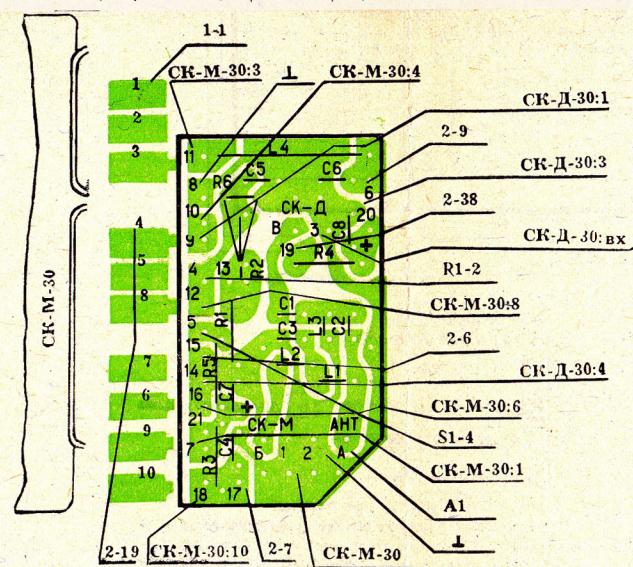
Плата 6.
