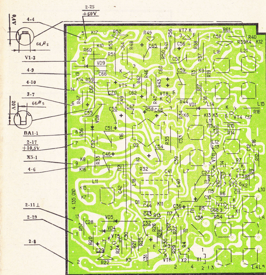
Плата 1. ФСС УПЧИ видеоусилитель, УПЧЗ УНЧ
