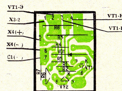
Плата 5. Плата стабилизатора
