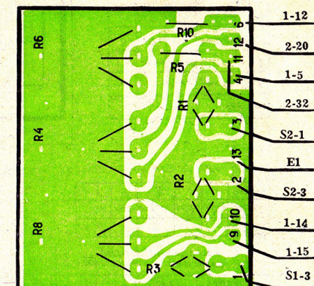
Плата 5. Плата стабилизатора
