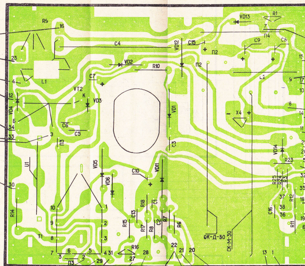
Плата 2. Выходной каскад строчной развертки, цепи питания кинескопа, селекторы каналов
