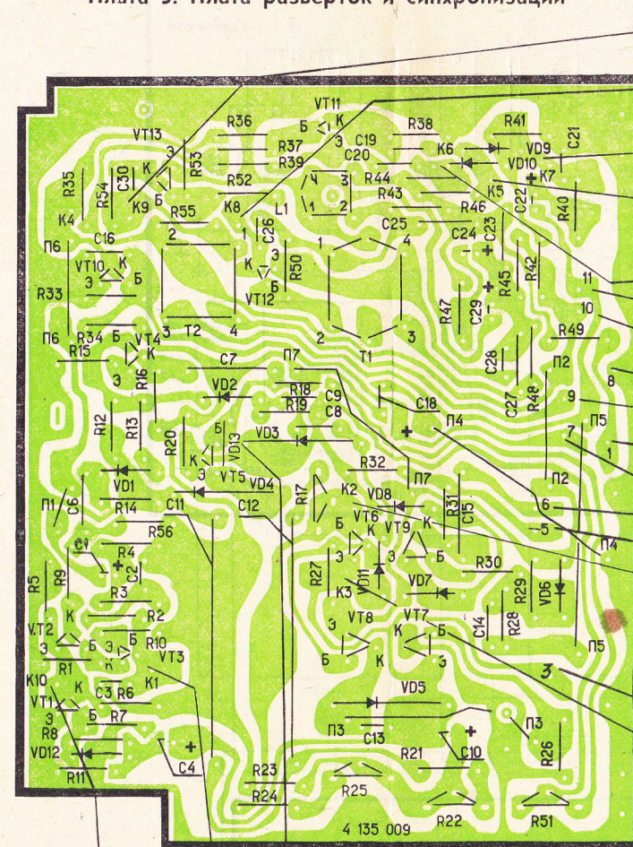
Плата 3. Плата разверток и синхронизации
