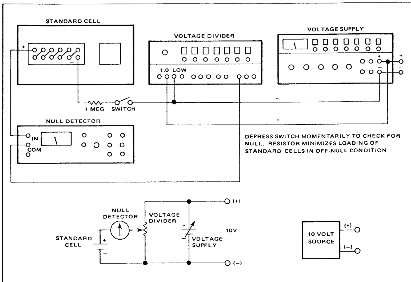
Figure 5.1 - 10 Volt Source
