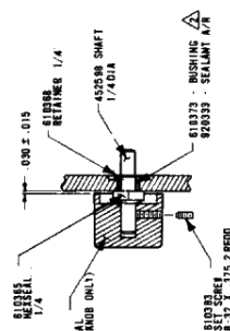
SECTION A-A SCALE: 1/1 TYPING RANGE & FUNCTION
