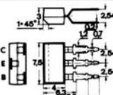
Bild 18 ≈ SOT-25
