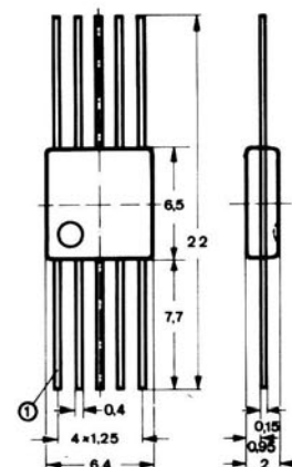
Kunststoffgehäuse \approx TO-91 Plastic case
