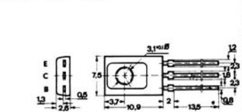
Bild 37 SOD-37
