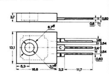
Bild 30 SOT-32
