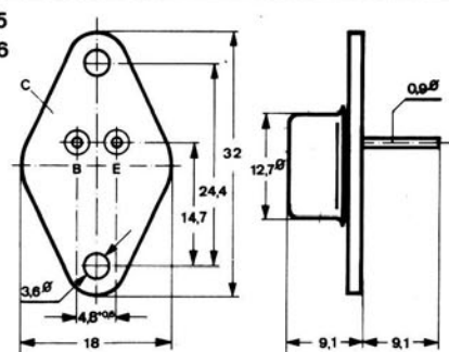
Bild 25 TO-66
