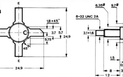
Bild 13 SOT 48
