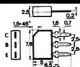
Bild 24 SOT-9
