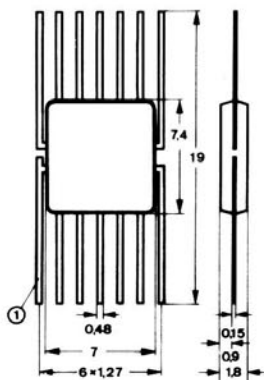
Keramik/Metallgehäuse TO-86 Ceramic/Metal case
