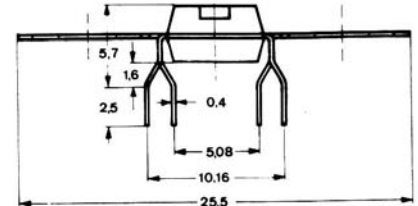
Metallgehäuse TO-96 Metal case
