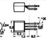
Bild 21 ≈ TO-92
