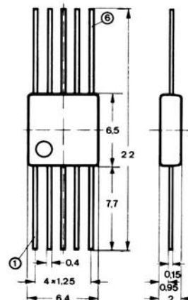
Keramik/Metallgehäuse ~ TO-91 Ceramic/Metal case
