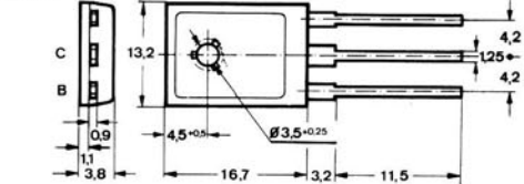
Bild 12 C 90
