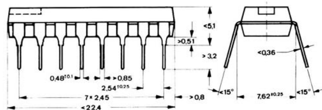
Kunststoffgehäuse TO-116 Plastic case
