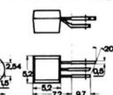
Bild 26 TOP-3
