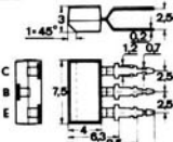
Bild 17 ≈ SOT-25
