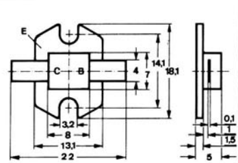
Bild 29 ≈ TOP-66
