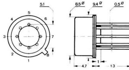
Metallgehäuse TO-99 Metal case
