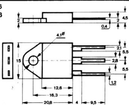
Bild 26 TOP-3
