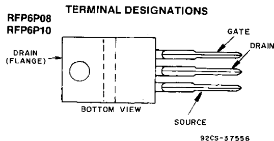
JEDEC TO-220AB
