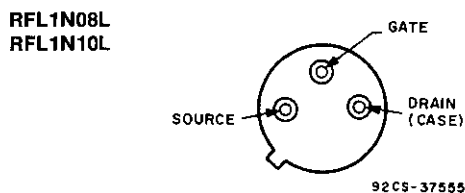
JEDEC TO-39
