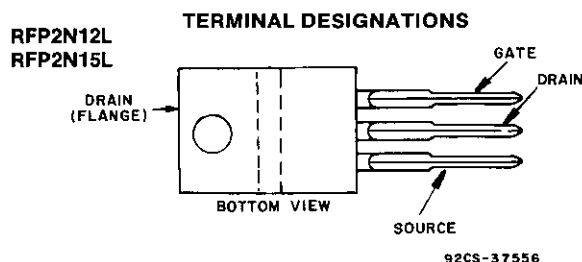
JEDEC TO-220AB
