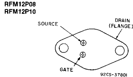
JEDEC TO-204MA
