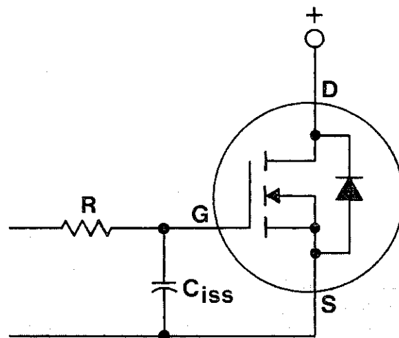
Basic power MOSFET input circuit.
