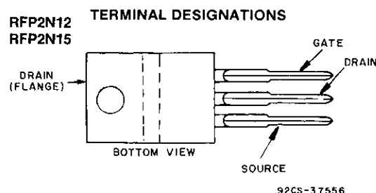
JEDEC TO-220AB
