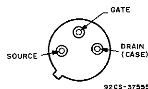
JEDEC TO-39
