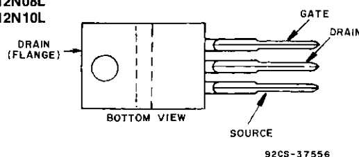
JEDEC TO-220AB
