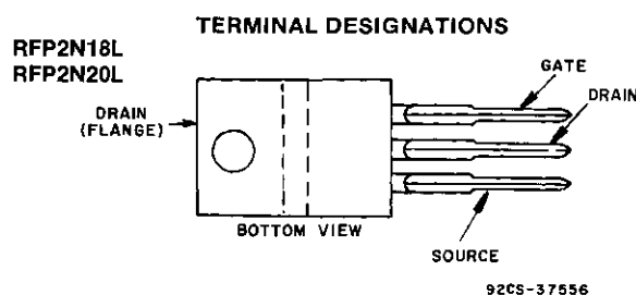
JEDEC TO-220AB
