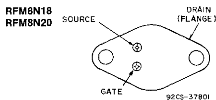
JEDEC TO-204MA
