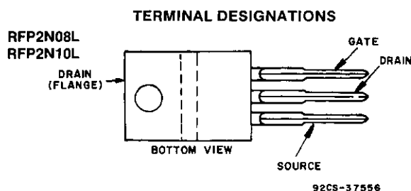
JEDEC TO-220AB
