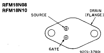
JEDEC TO-204MA
