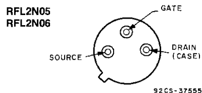
JEDEC TO-39
