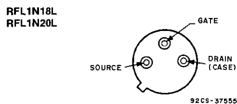
JEDEC TO-39
