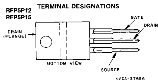
JEDEC TO-220AB
