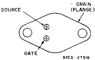
JEDEC TO-204AE
