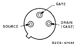
JEDEC TO-39
