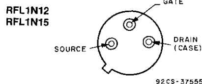
JEDEC TO-39
