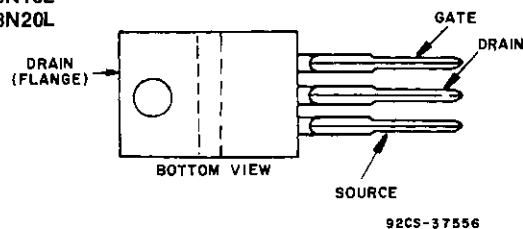
JEDEC TO-220AB
