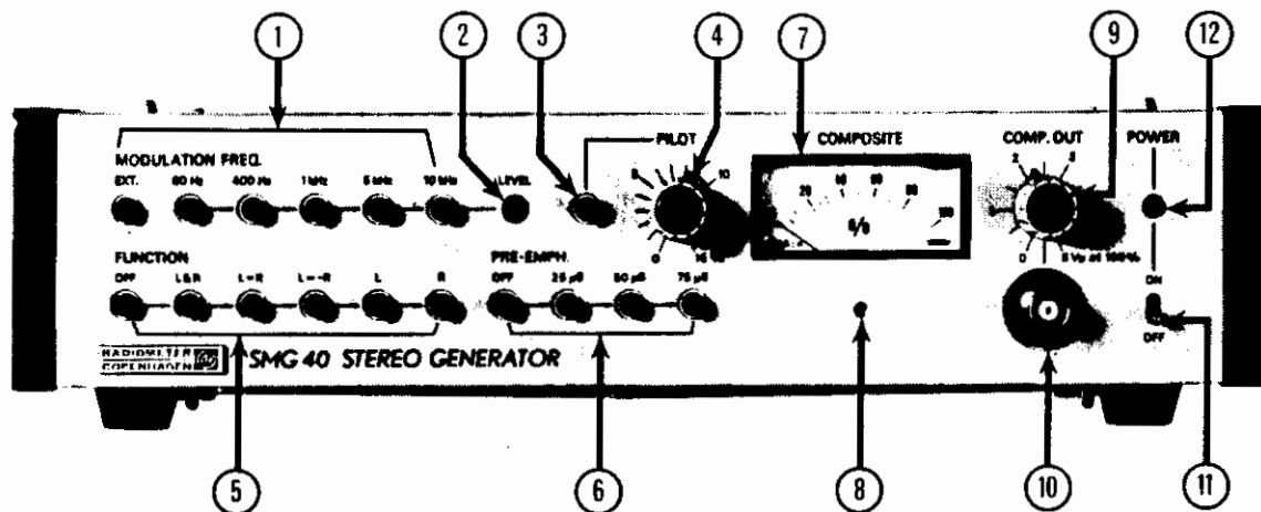
FIG. B1
