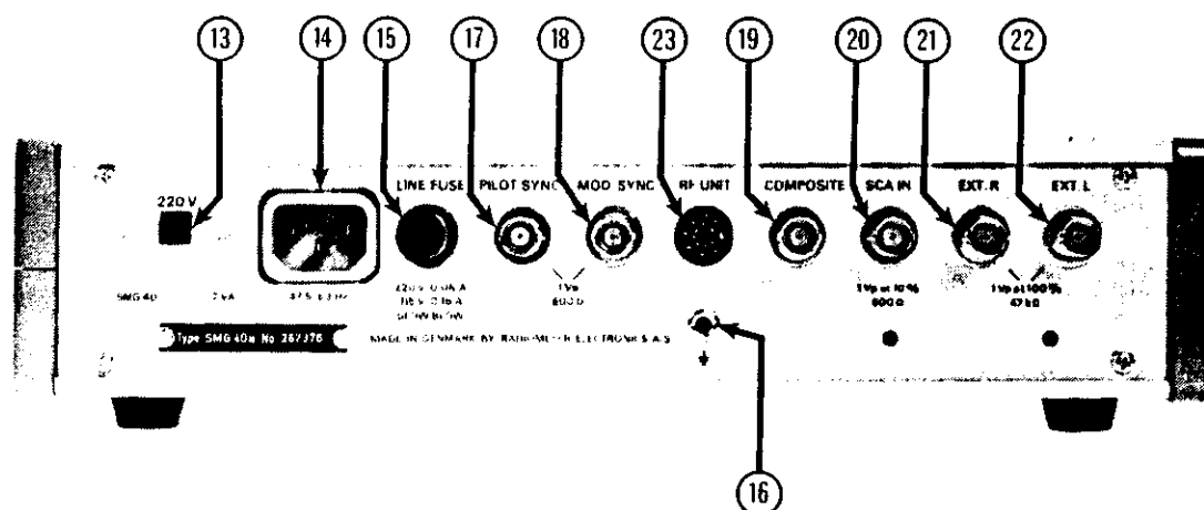
FIG. B 2
