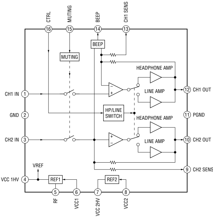
IC381 AN17020A-VB
