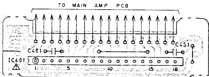
POWER IC PCB C1036A501D
