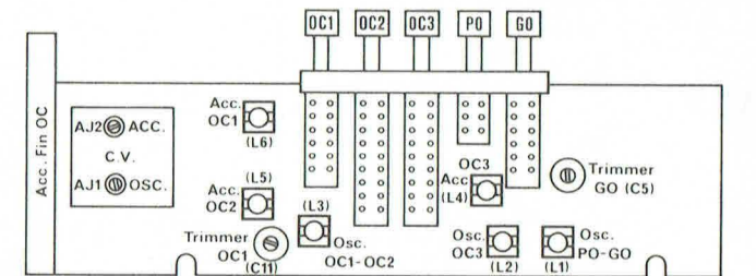
EMPLACEMENT DES RÉGLAGES SUR LE CIRCUIT H.F.
