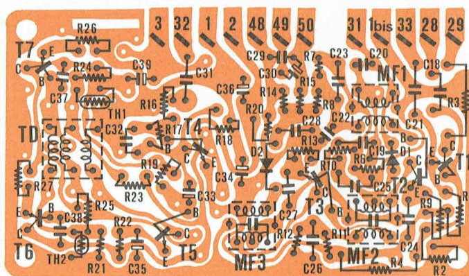
FI + BF COTÉ CUIVRE
