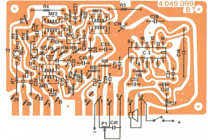
HF COTÉ ÉLÉMENTS
