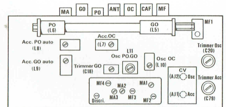
EMPLACEMENT DES RÉGLAGES
