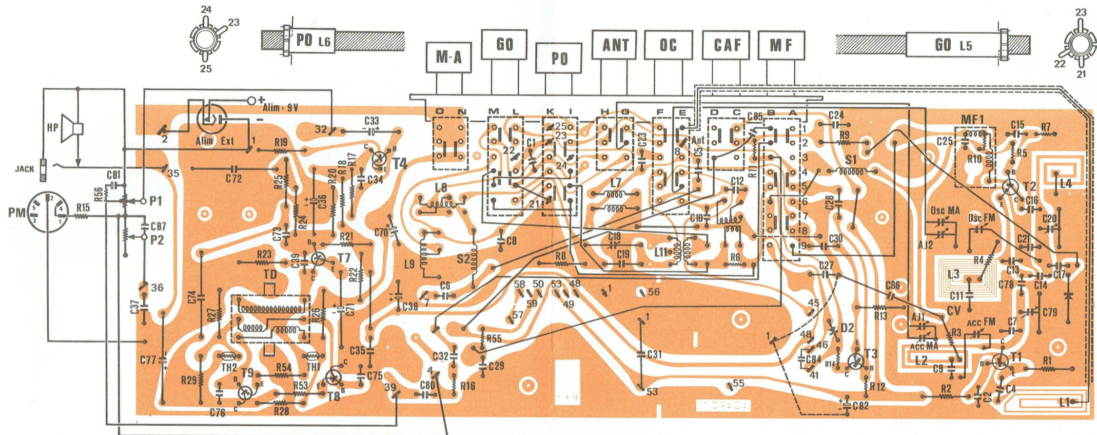
VU COTÉ ÉLÉMENTS
