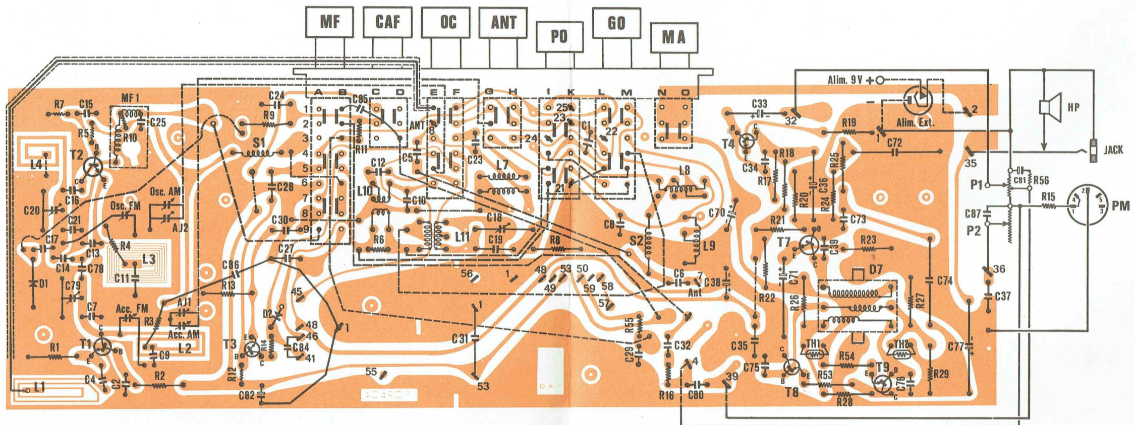
VU COTÉ CUIVRE
