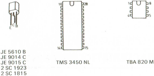
BROCHAGE DES SEMI-CONDUCTEURS
