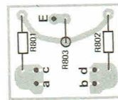
PLATINE ALIMENTATION SECTEUR (côté éléments)
