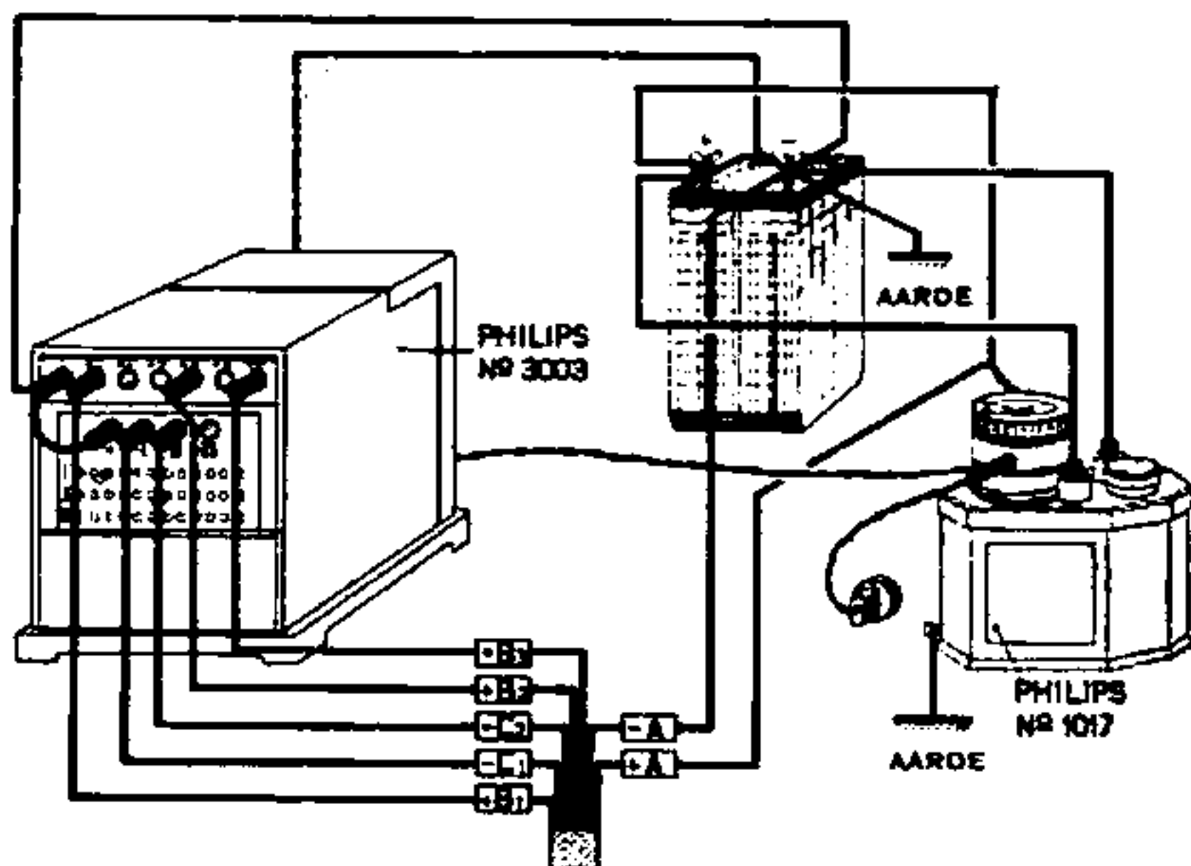
Fig. 3 Bij gebruik van Philips plaatspanningsapparaat No. 3003 en Philips gelijkrichter No. 1017 (De neg. roosterspanning van bus -I is op -4 V, van bus -II op -15 V ingesteld)
