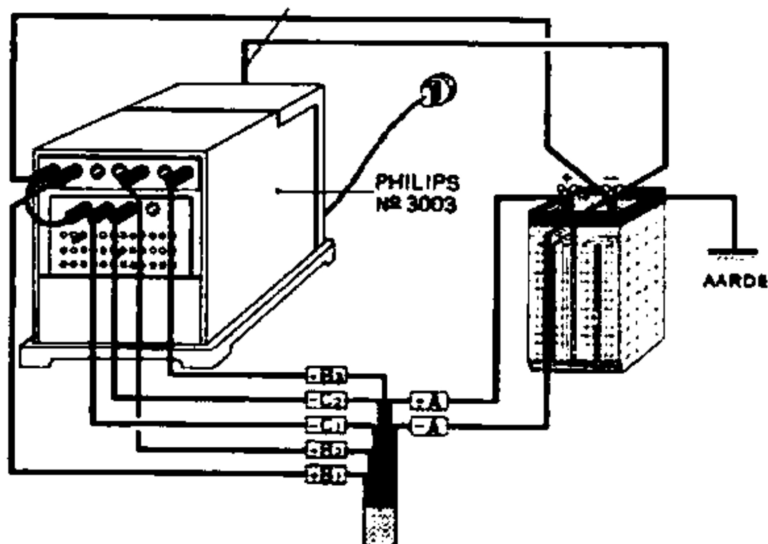
Fig. 4 Bij gebruik van Philips plaatspanningsapparaat No. 3003 (De neg. roosterspanning van bus -I is op -4 V, van bus -II op -15 V ingesteld)
