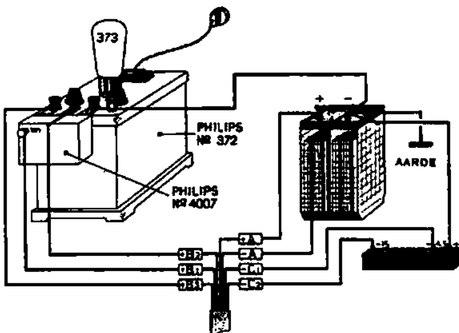
Fig. 6 Bij gebruik van Philips plaatspanningapparaat No. 372 („VOLT“-knop op stand „MAX“, „DET“-knop op stand III) met voorzetapparaat No. 4007 en met een batterij voor negatieve roosterspanning
