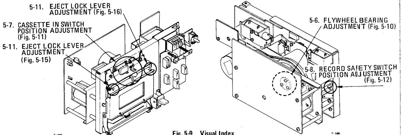
Fig. 5-9 Visual Index
