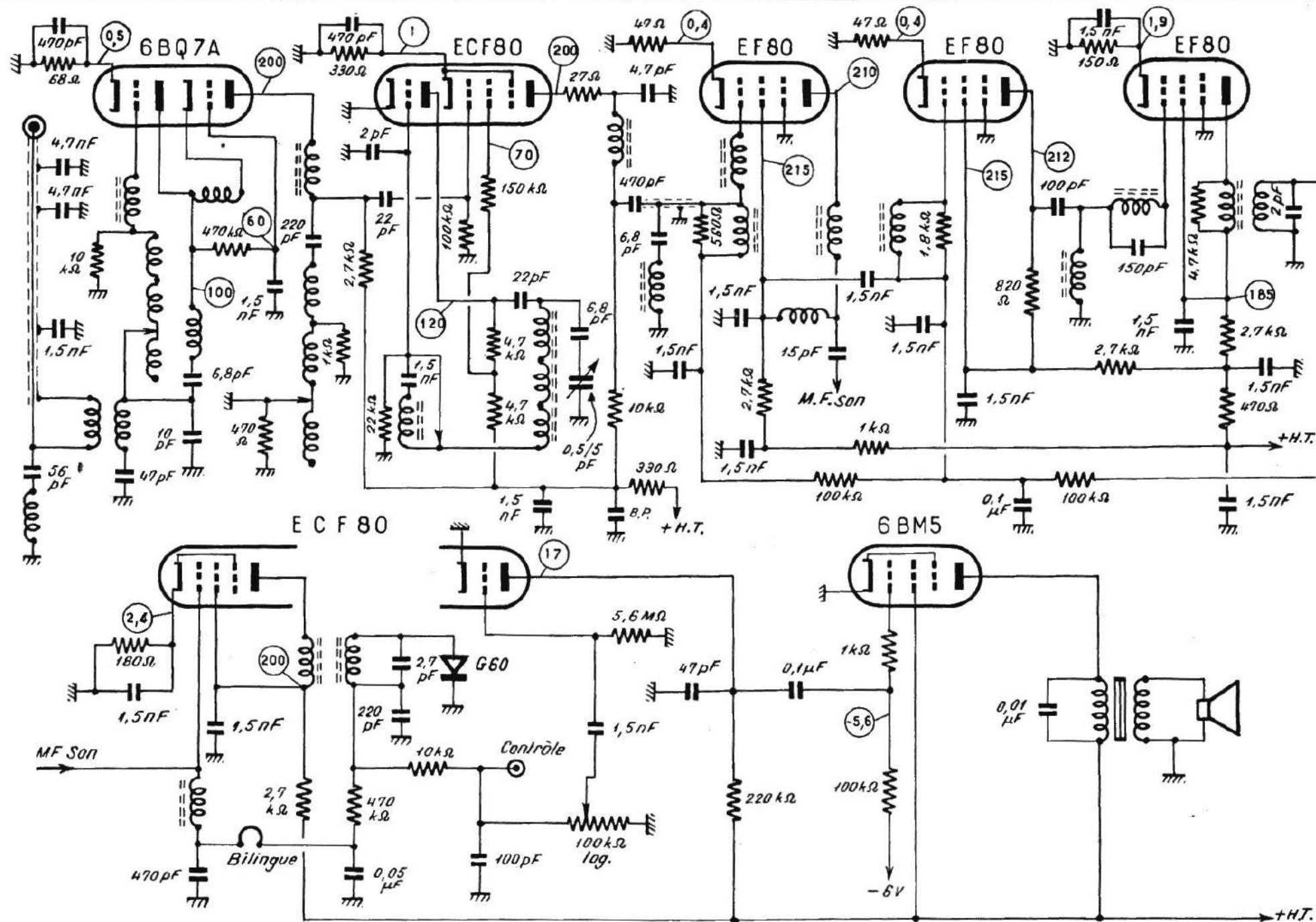
Etages H.F. et changement de fréquence, amplificateur M.F. vision, et récepteur son.
