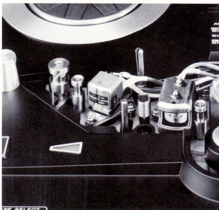
TC-850-2 Stereo-Tonbandgerät in Halbleitertechnik
