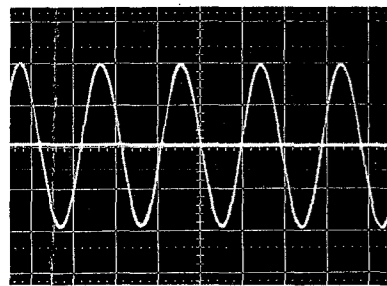
1 X = 5 \mu s/Skt.; Y = 0,02 V/Skt.
