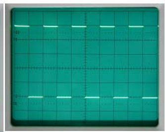
2 : 1 correct
