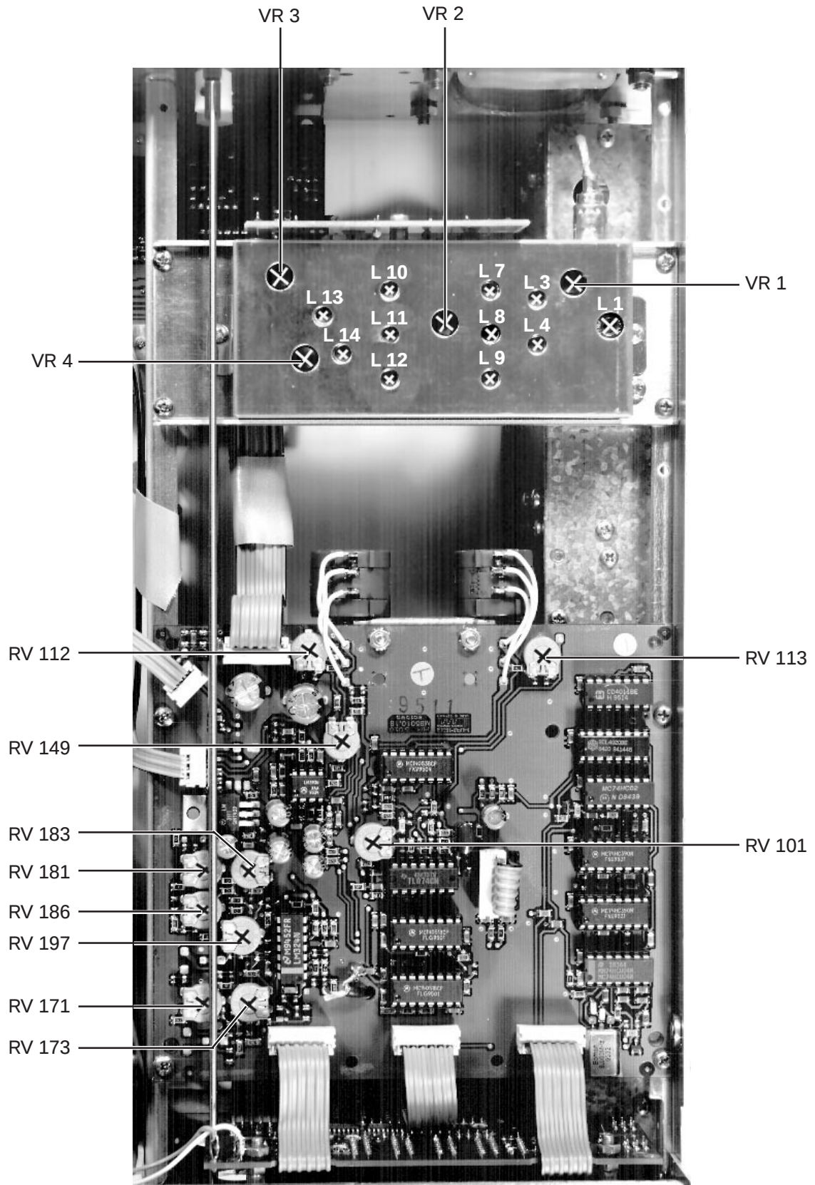
Bild 3 - Main-Board
