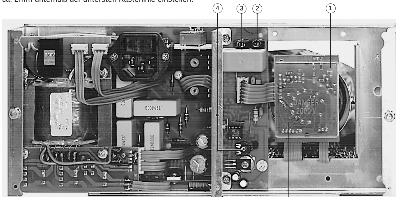
Bild 1. PS-Board
