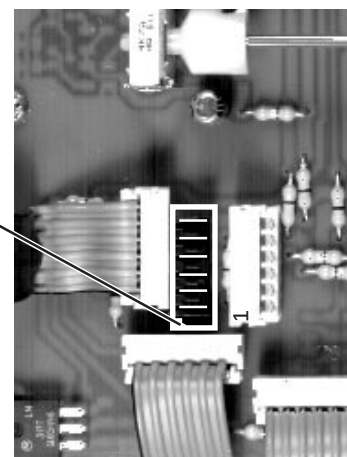
Bild 2. XYF-Board (Teil)
