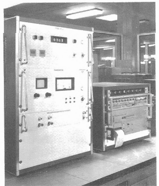
Ensemble " Générateur-Synthétiseur CS 201 + Programmateur 211 + Afficheur 221 " incorporé dans un système de contrôle automatique de filtres (Société anonyme des télécommunications - S.A.T. - France).
