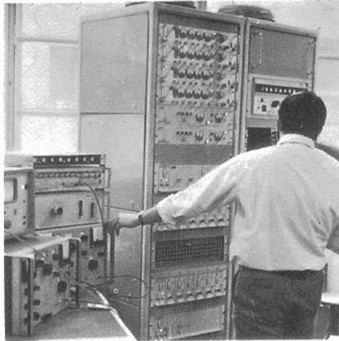
Utilisation d'un ensemble " Générateur-Synthétiseur 2 MHz - CS 201 + Programmateur IRIG (T) 290 + Afficheur 221 " pour le contrôle d'une baie de télémesures FM/FM (Nord-Aviation - France)
