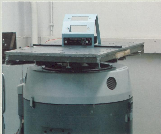
Rütteltisch
