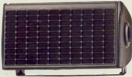
EN 8355 Breitbandsystem mit Hochtonkegel Belastbarkeit 20 Watt Übertragungsbereich 150-18 000 Hz
