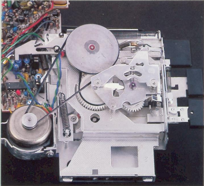
Philips-Cassettenlaufwerk
