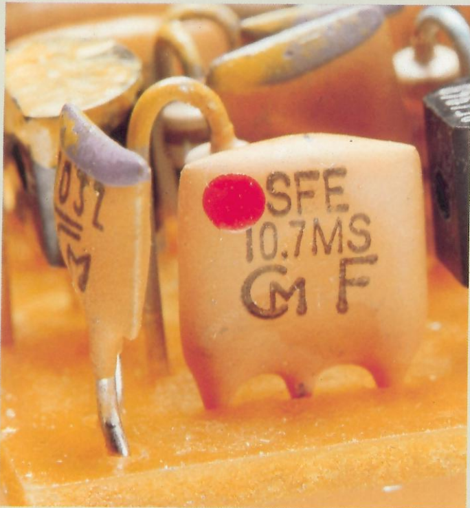
Keramikfilter
