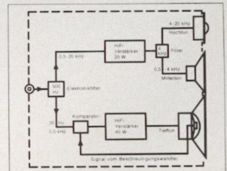
Die MFB-Box RH 532 im schematischen Aufriß: 3-Weg-Box mit 2 integrierten Verstärkern für Mittel-/Hochton und Tiefton mit PXE-Wandler.
