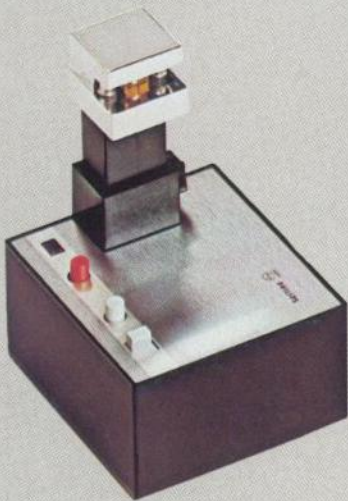
N 6400 Dia-Steuergerät zur Steuerung automatischer Dia-Projektoren. Für alle Tonbandgeräte. Impulsiage auf Spur 4. Impulsfrequenz ca. 1000 Hz. Transistorisiert. Batteriebetrieb (mehr als 100 Std. Betriebsdauer). Anschluß für Netzvorsichtgerät (7,5 V). Drucktastensteuerung. Löschanzeige. Impulslöschung. Höhenverstellung. DM 145,-*
