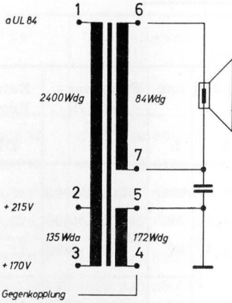
Schaltung
