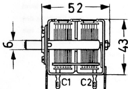
Zweifach-Drehkondensator
