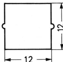
Chassisdurchbruch
