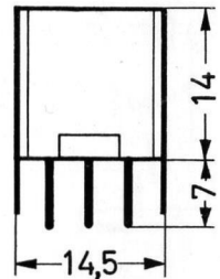
Maßskizzen
