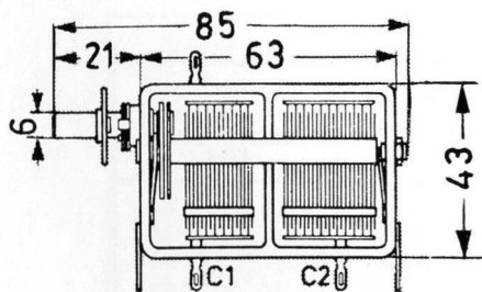
Zweifach-Drehkondensator
