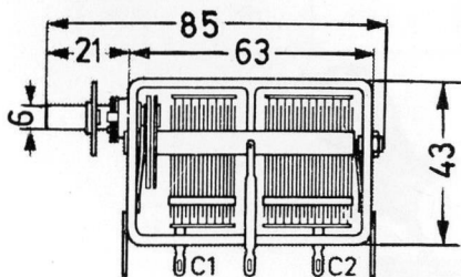
Zweifach-Drehkondensator
