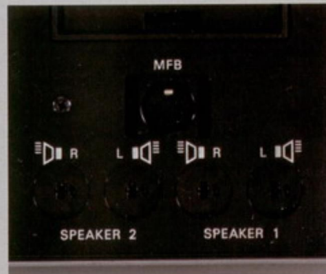
Uitgangen voor 2 stereo luidsprekersystemen. Dus moge- lijkheid voor o.a. Stereo-4. Bovendien 1-volt aansluiting voor MFB boxen.
