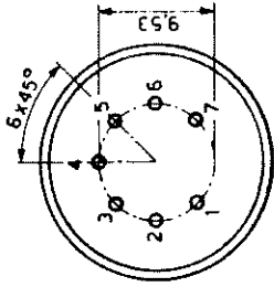
MINIATURA a 7 piedini
