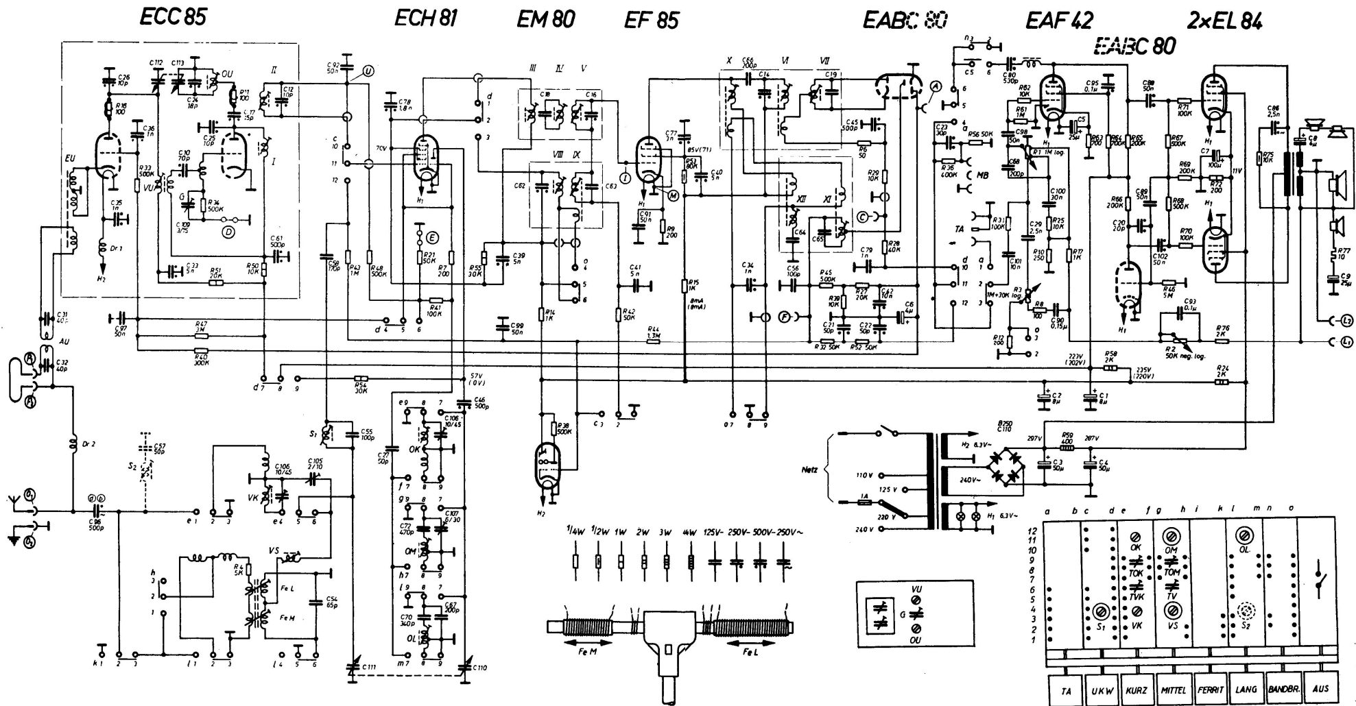
METZ RADIO APPARATEFABRIK (Capriotti) - Mod. AM/FM 405 3D/WF. A modulazione d'ampiezza e di frequenza. Onde medie lunghe corte e ultracorte (FM). Media frequenza AM a 460 kc/s, e FM a 10,7 Mc/s. Riproduzione stereofonica con quattro altoparlanti. Potenza d'uscita 8 watt indistorti. Consumo 68 watt.
