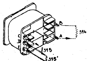
Transfo. déphaseur : FD 041 10
