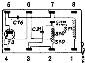
Filtre MF 3 : FD 002 29
