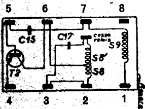
Filtre MF 2 : FD 002 27
