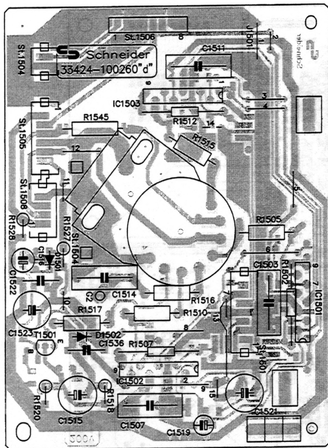
(16:9) Bestückungsseite/Top view
