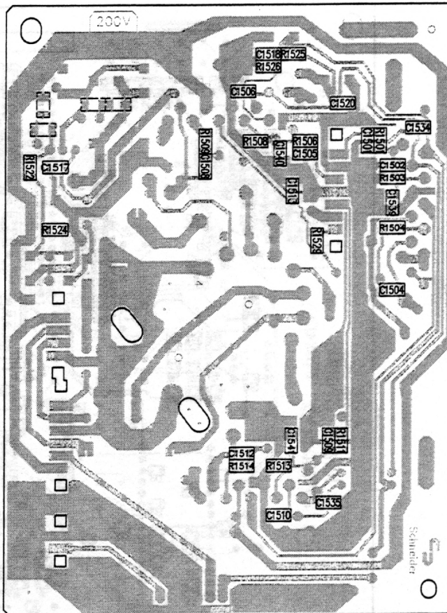
Chip-Seite/Bottom view
