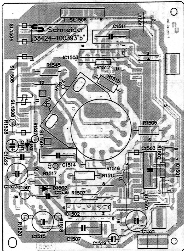
(16:9) Bestückungsseite/Top view
