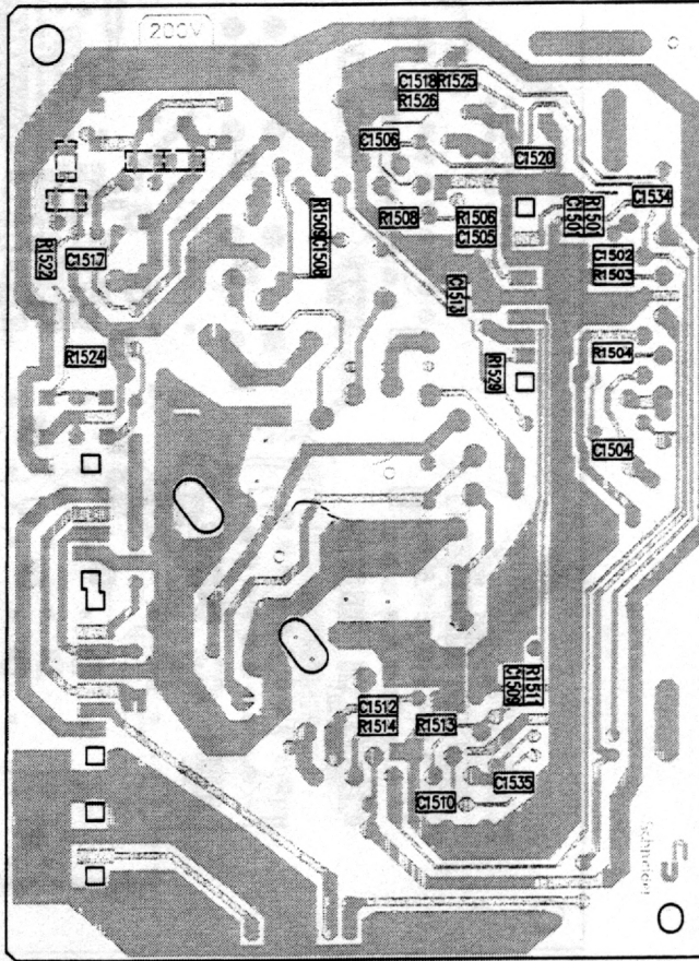
Chip-Seite/Bottom view
