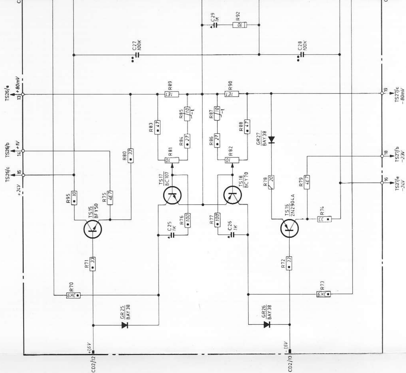
Fig. 27. Schéma de principe de l'amplificateur de puissance
