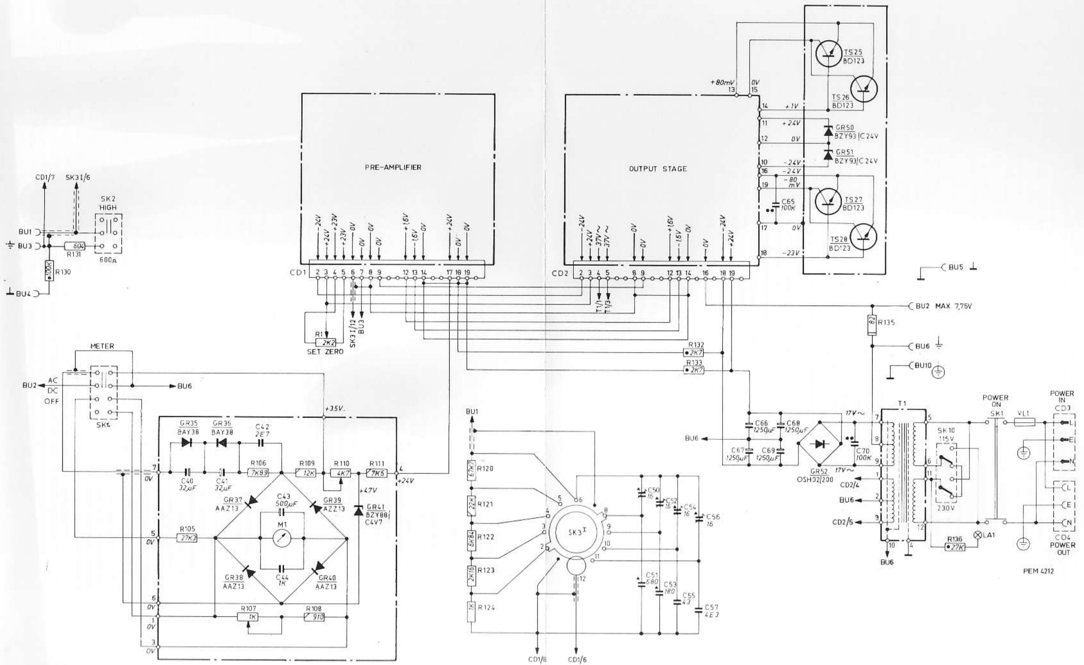
Fig. 28. Schéma de principe général
