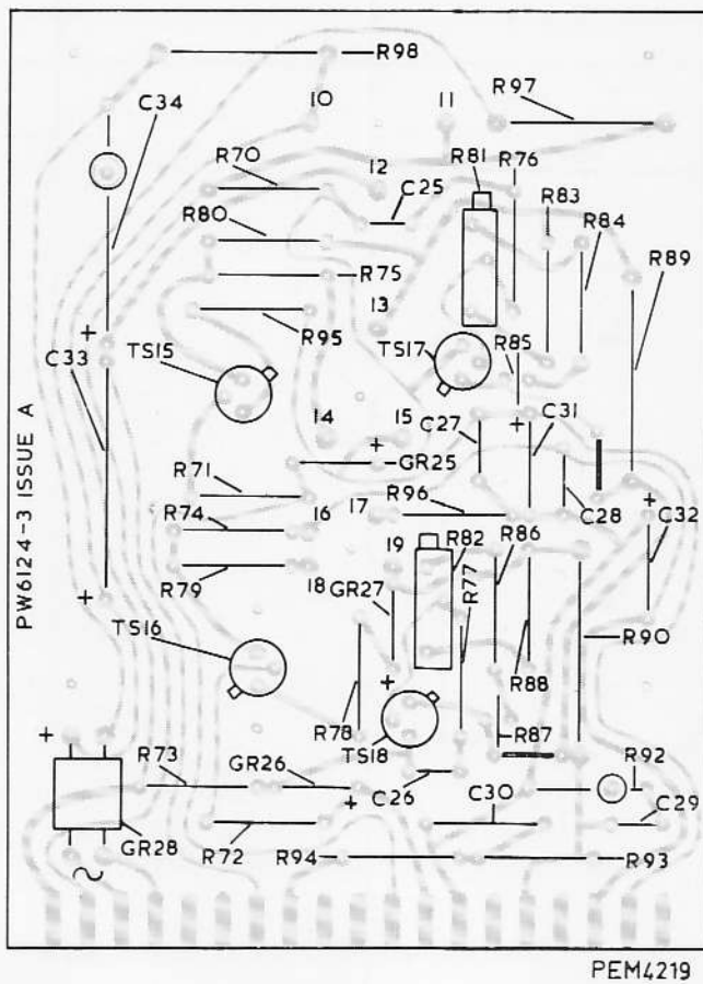
Fig. 25. Platine imprimée de l'amplificateur de puissance
