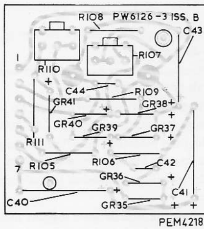
Fig. 23. Platine imprimée du circuit du voltmètre
