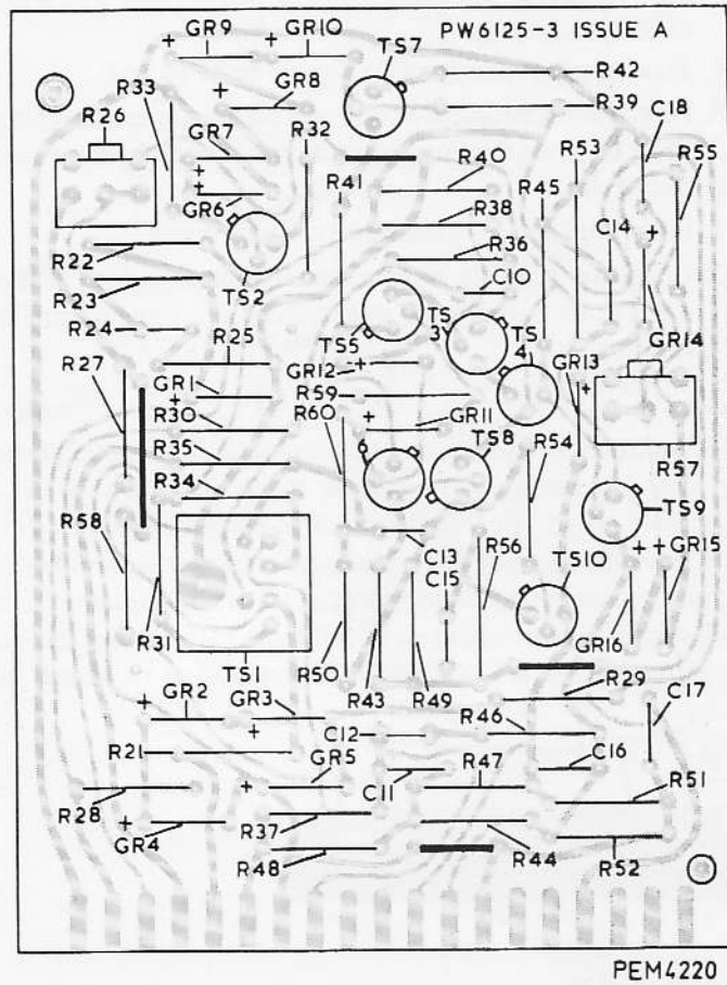
Fig. 24. Platine imprimée du préamplificateur
