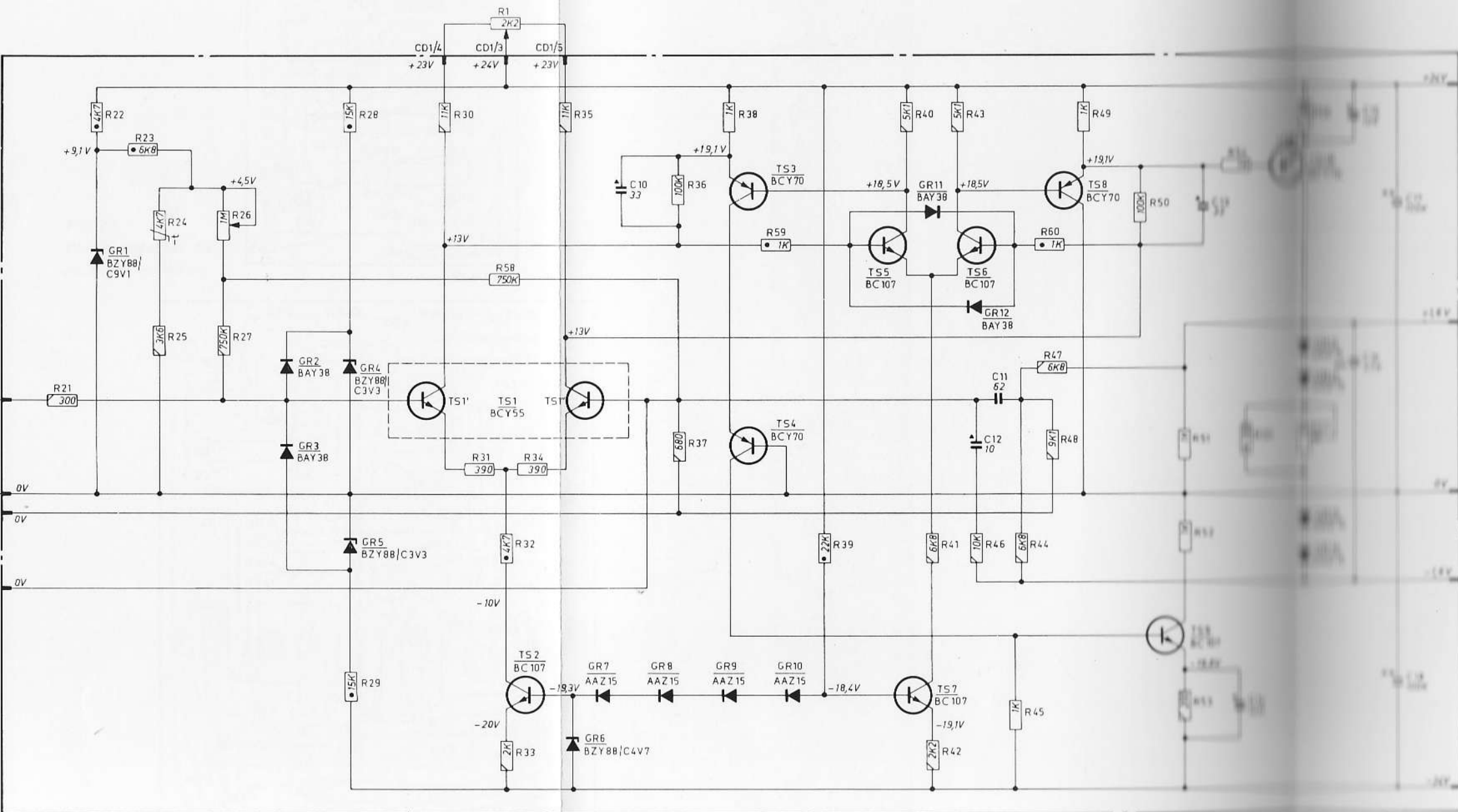
Fig. 26. Schéma de principe du préamplificateur
