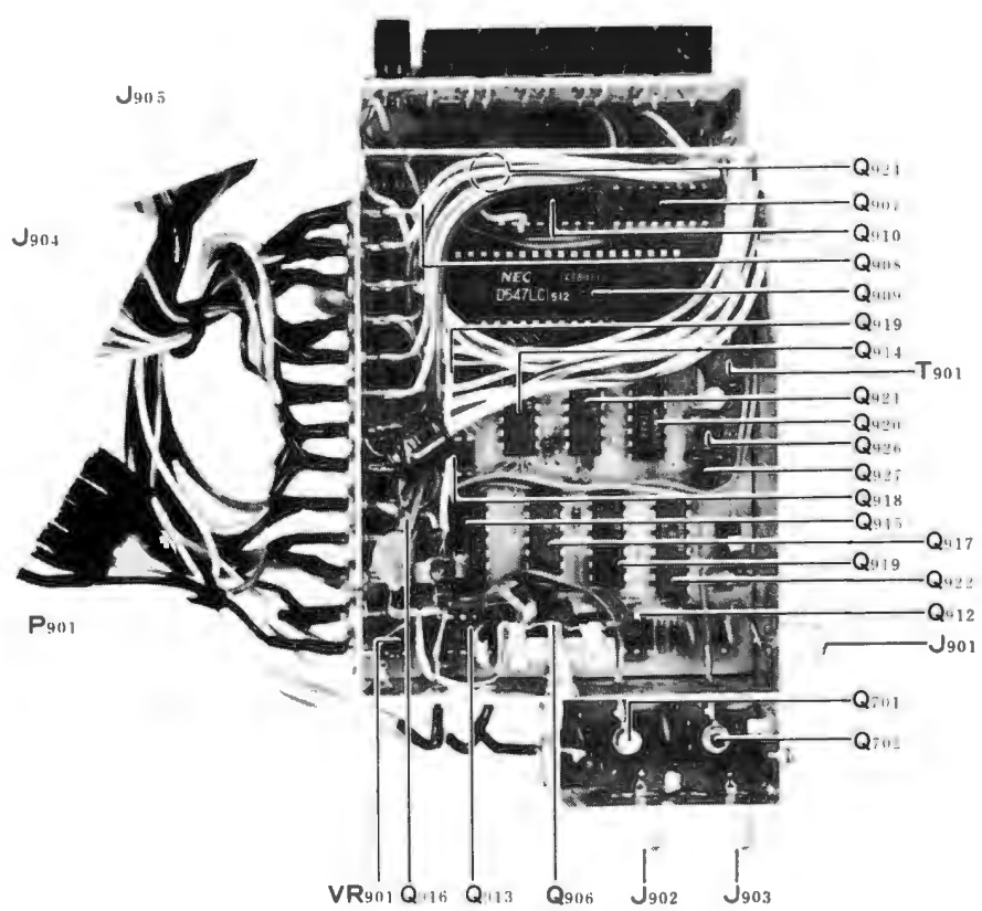
COUNTER UNIT(PB-1754)
