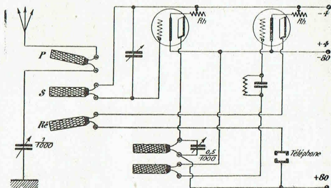
11. — Une Lampe H. F. à transfo accordé, une détectrice .
