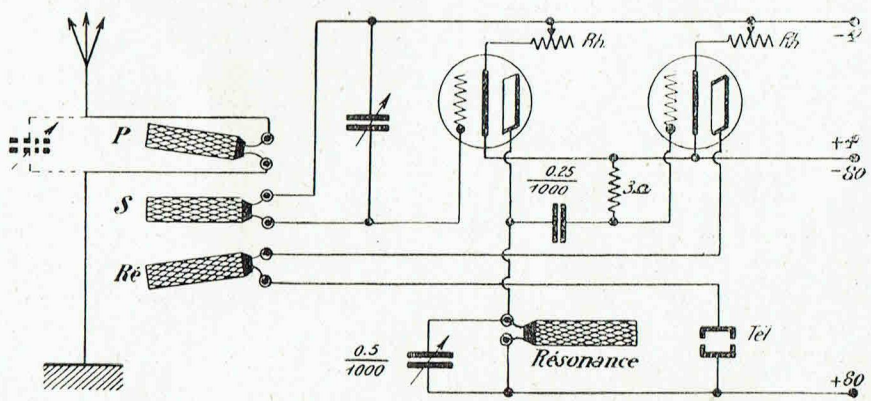
9. -- Une Lampe H. F. à résonance, une détectrice.
