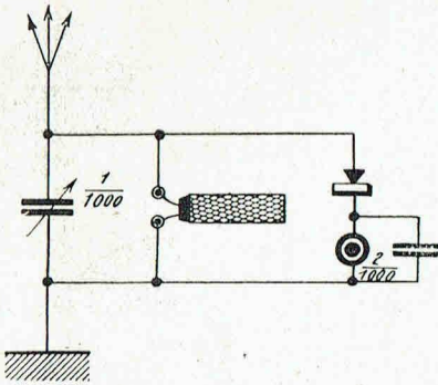
1. — Galène, accord en direct.
