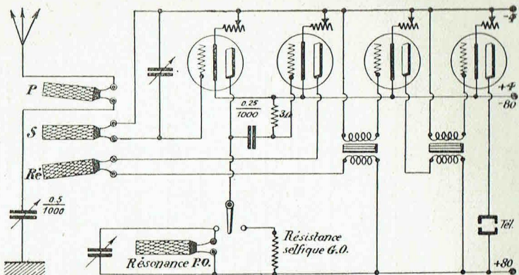
10. — Une Lampe H. F. pour petites et grandes ondes, une lampe détectrice , 2 B. F. à transfo.
