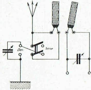
4. — Système d'accord tesla, condensateur primaire, série ou dérivation.
