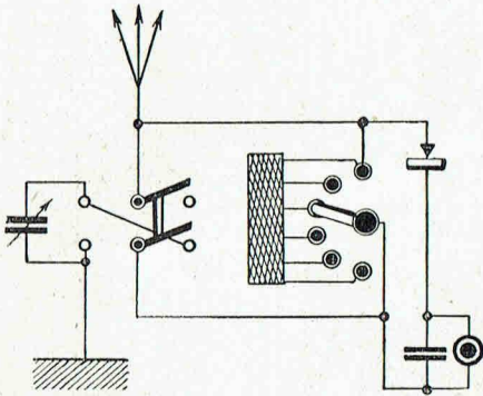
3. — Galène, accord en direct par bobine fractionnée.
