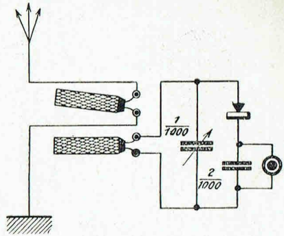
2. — Galène, accord en tesla.
