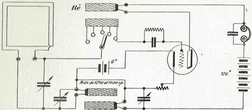
13. — Super-Réaction sur cadre.
