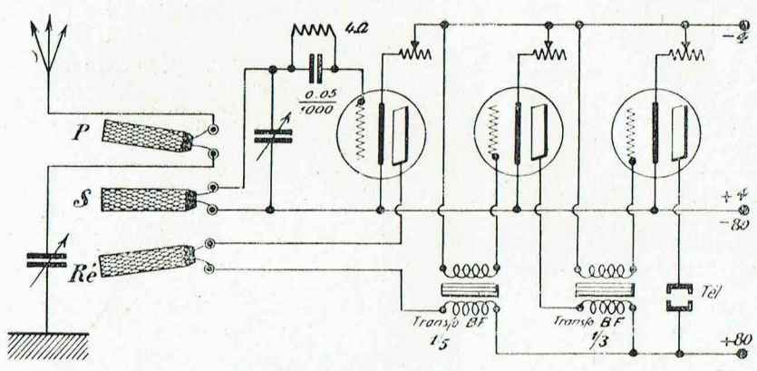
8. -- Lampe détectrice suivie de 2 B. F. à transfos.
