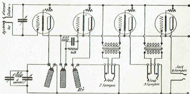
12. — Amplificateur à combinaisons, réaction sur le transfo accordé, évitant ainsi les radiations dans l'antenne (ce système peut également s'appliquer aux schémas 9, 10 et 11).
