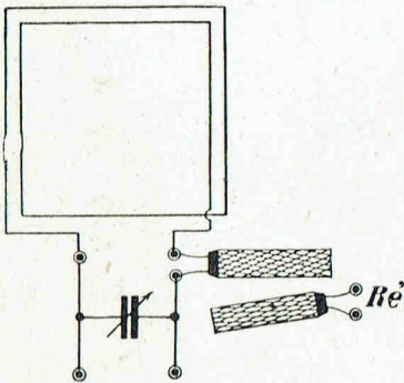
5. — Réaction sur cadre
