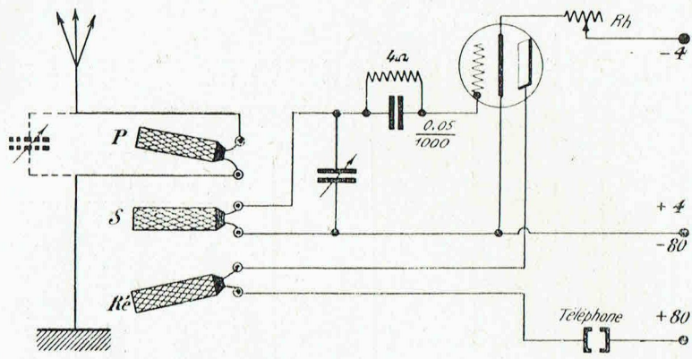
7. -- Lampe détectrice à réaction avec accord
