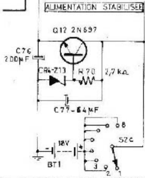
MESUREUR DE CHAMP VX403A METRIX
