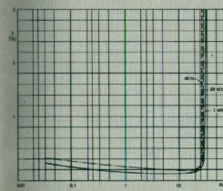
Klirrfaktor
