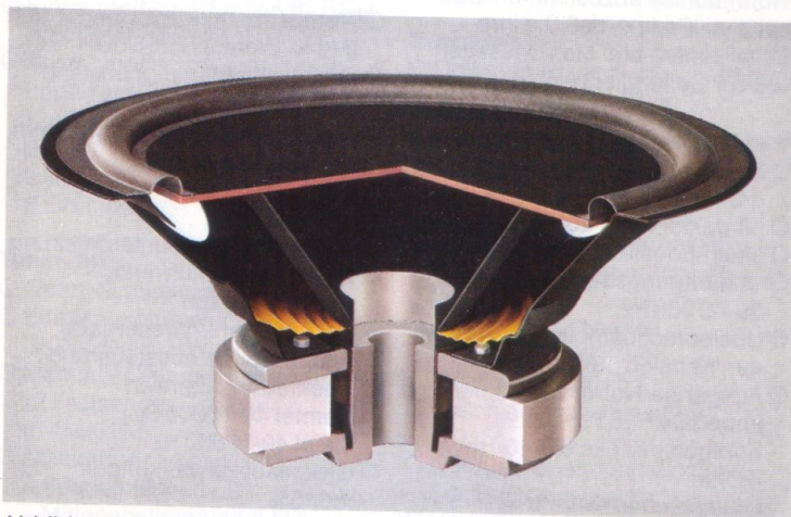
Abbildung oben: Querschnitt durch den Tieftöner in Glasfaser-Flachmembran-Technik.
