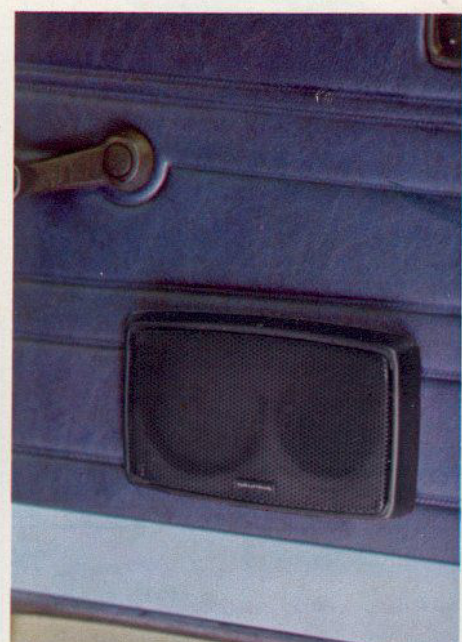
Einbaulautsprecher L/U 80 Nennbelastbarkeit 20 W Musikbelastbarkeit 30 W Übertragungsbereich 63... 20000 Hz Maße: ca. 205 × 33 × 125 mm; zusätzlich 58 mm für Einbautiefe erforderlich. Geschlossene Zweiweg-Box! Lieferbar Sommer 1980
