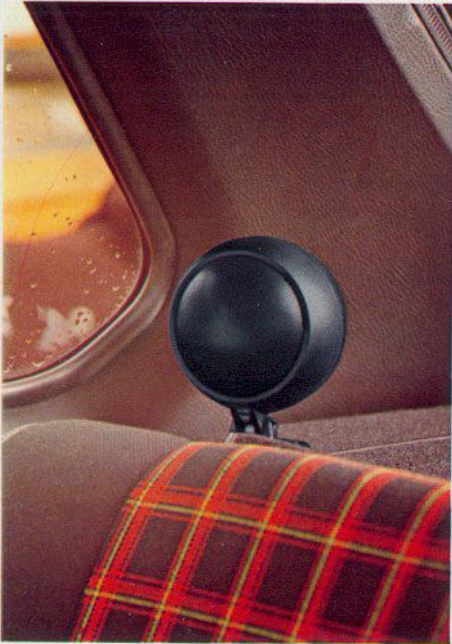
Kugellautsprecher L/U 18 mit verstellbarem Abstrahlwinkel! Nennbelastbarkeit 15 W Musikbelastbarkeit 25 W Übertragungsbereich 100... 12500 Hz Höhe mit Fuß = ca. 148 mm, Kugeldurchmesser = ca. 118 mm.
