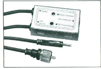
Antennenweiche Moba 9010 Für Antennen Moba 9000 und Moba 3500 für CB-Sprechfunk und gleichzeitigen Rundfunkempfang.
