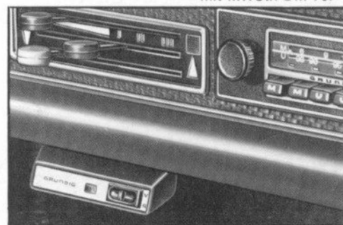
Verkehrs-Rundfunk-Decoder VD 2 Für Montage unter dem Armaturenbrett. Befes- tigung mit 2 Schraubtaschen. Funktionen im Prinzip wie bei VD 1. Abmessungen: 114 x 35 x 70 mm (B x H x T) unverbindliche Preisempfehlung mit MWSt.: DM 60.-
